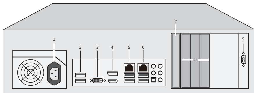
图1-3 TL-VMS616后面板示意图
