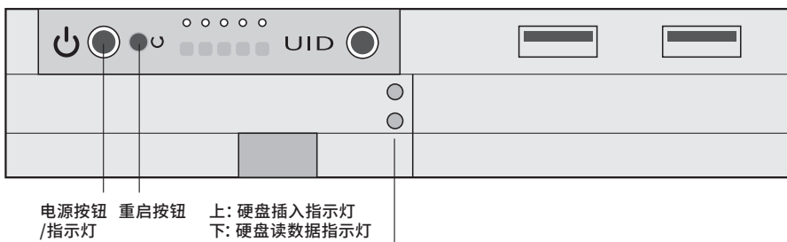
图1-2 前面板按钮与指示灯
